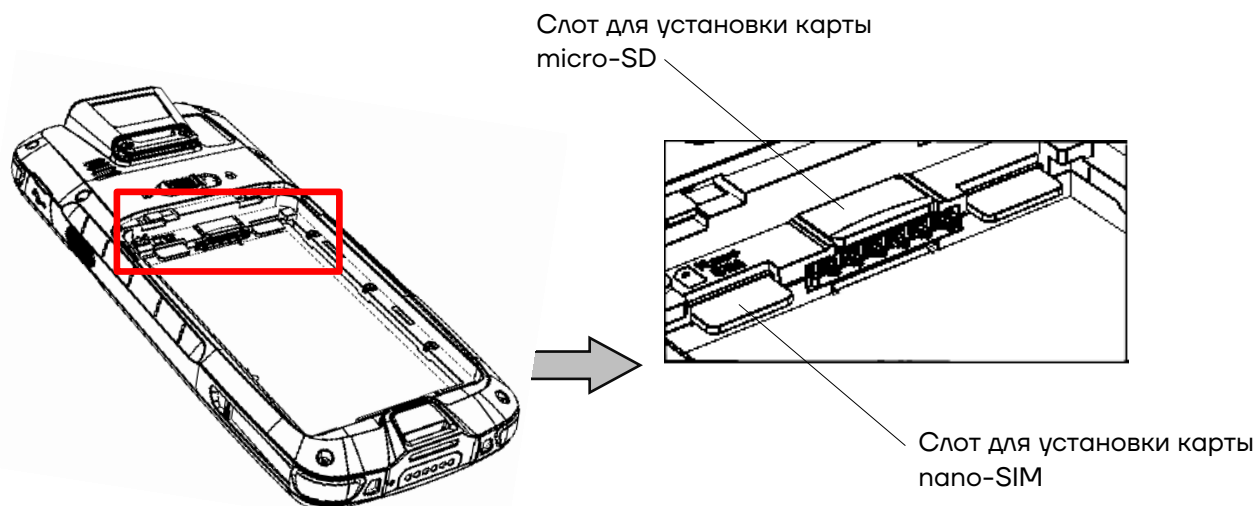
Рисунок 8. Расположение слотов для карт nano-SIM и micro-SD
