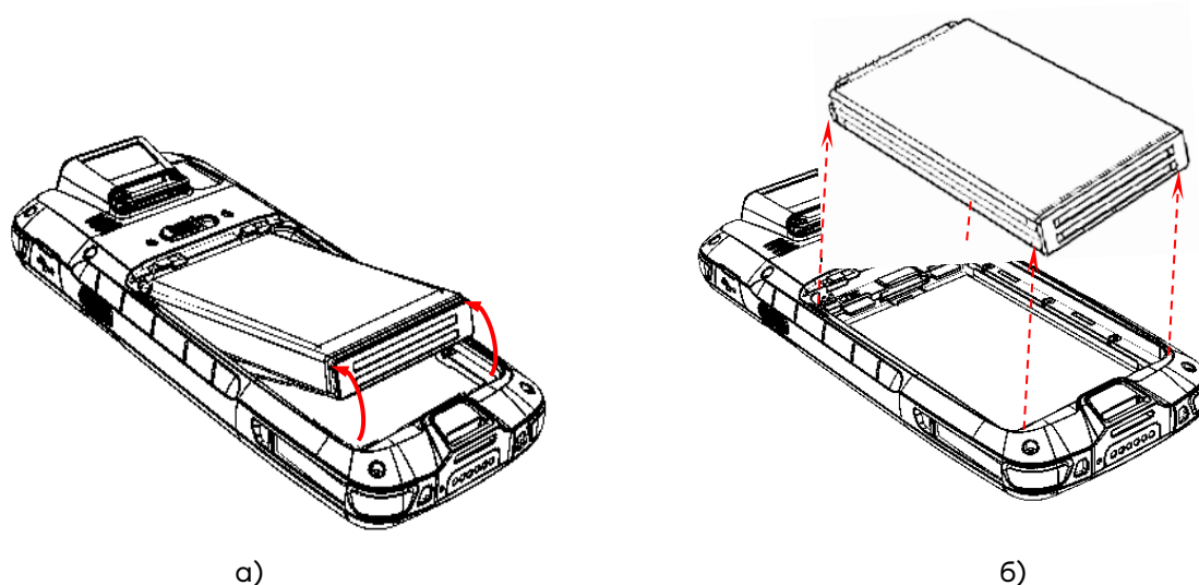
Рисунок 6. Извлечение аккумулятора: а) отделить нижнюю часть АКБ; б) извлечь АКБ
